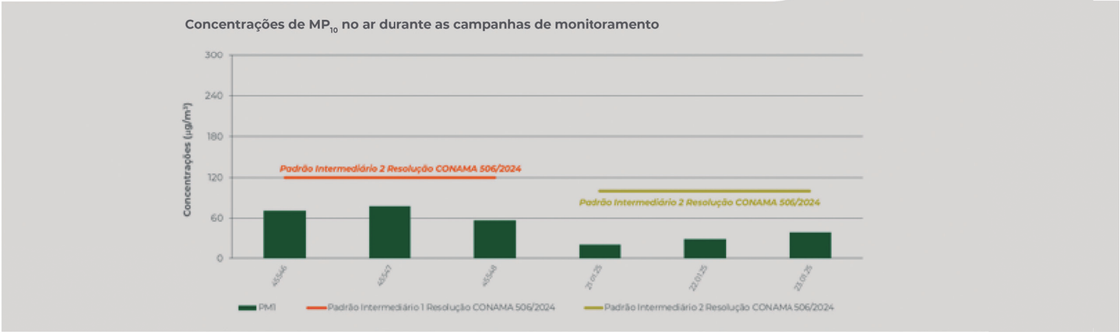
FIGURA 5.1.11.2 Concentrações de MP10 obtidas nas campanhas de monitoramento da qualidade do ar realizadas em setembro de 2024 e janeiro de 2025 na UMI.
