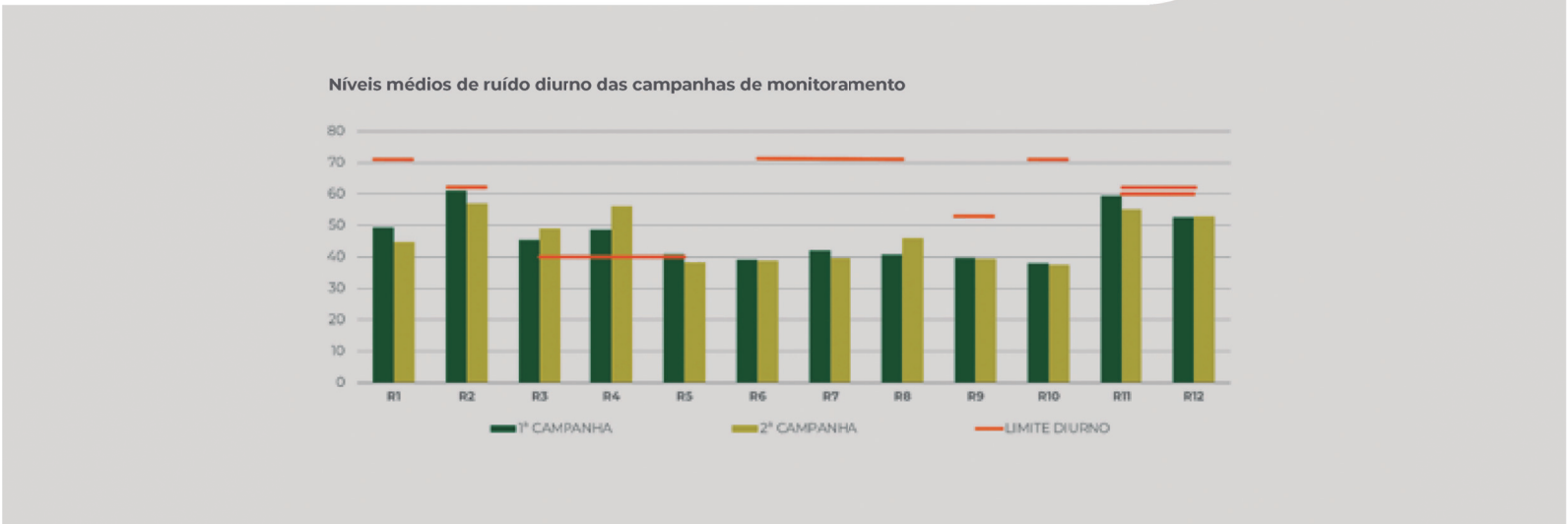
FIGURA 5.1.12.1 Níveis de ruído diurno registrados no entorno da área de interesse nas campanhas de monitoramento realizadas em setembro de 2024 e janeiro de 2025.
