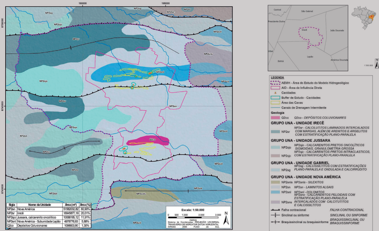
FIGURA 5.1.7.1 Área do Estudo do Modelo Hidrogeológico.
