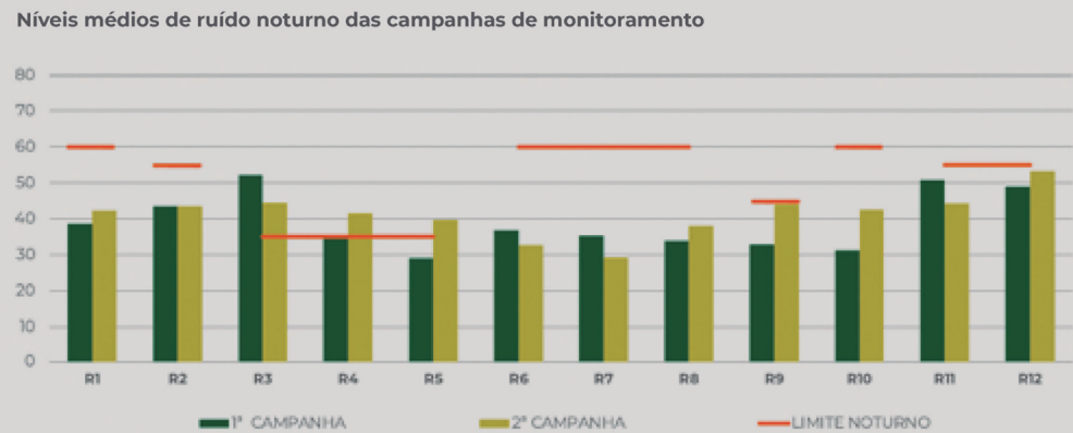
FIGURA 5.1.12.1 Níveis de ruído diurno registrados no entorno da área de interesse nas campanhas de monitoramento realizadas em setembro de 2024 e janeiro de 2025.
