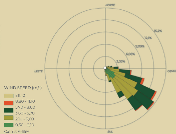
FIGURA: 5.1.4.6 Rosa dos ventos Irecê/BA (2008-2024). Fonte: INMET (2025).
