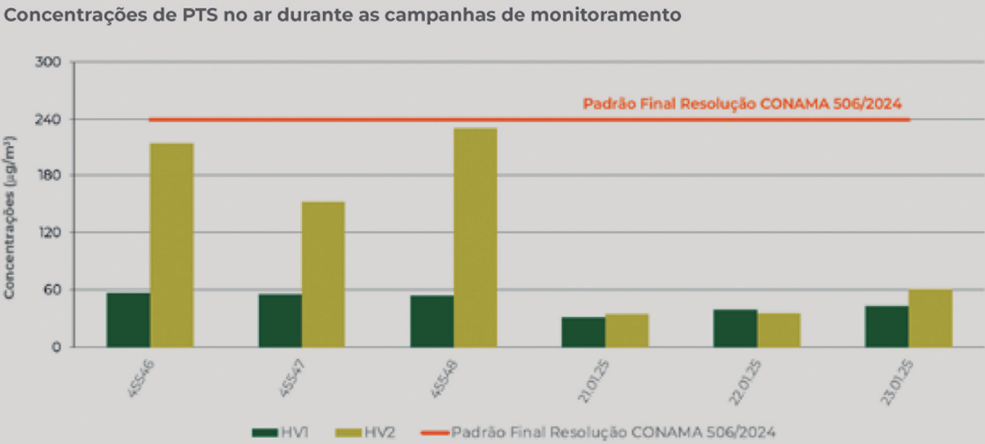
FIGURA 5.1.11.1 Concentrações de PTS obtidas nas campanhas de monitoramento da qualidade do ar realizadas em setembro de 2024 e janeiro de 2025 na UMI.
