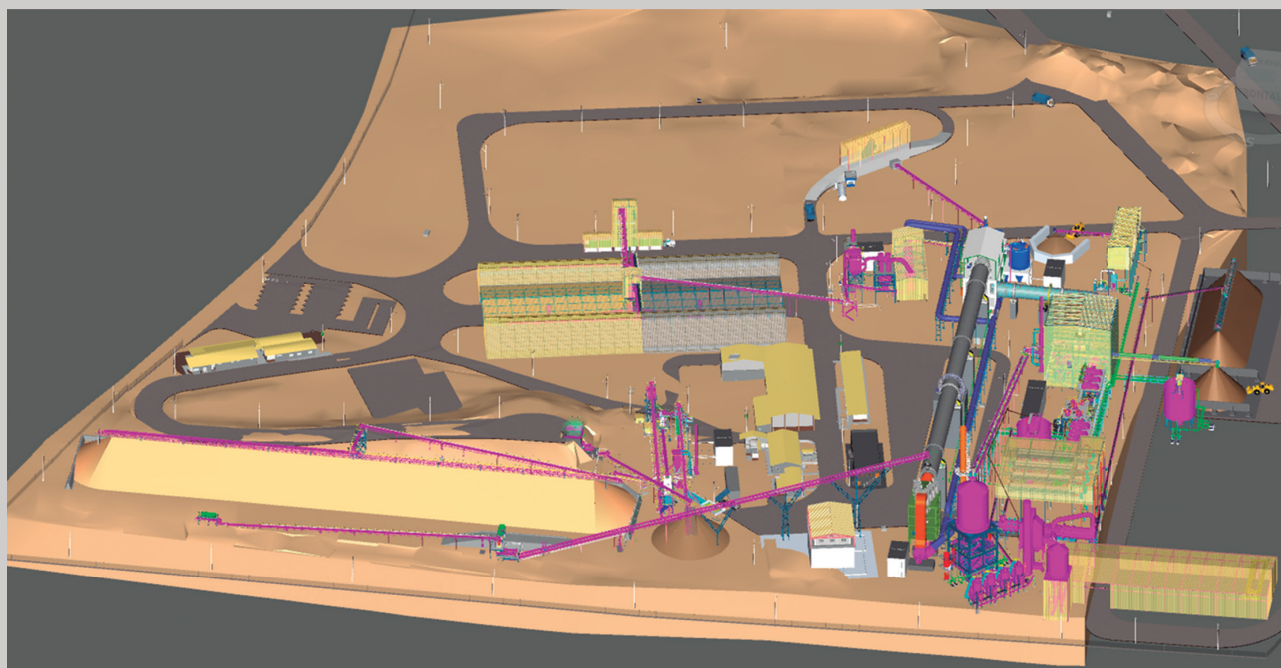
FIGURA 3.8.1.2 Vista oblíqua, de sul para norte, do modelo em 3D da futura área industrial da UMI da FOSNOR.
